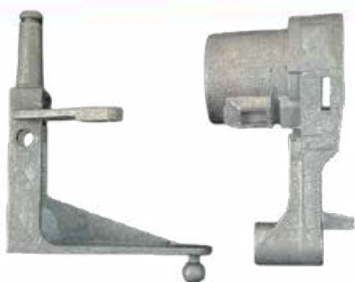
CÓD 289939 - KIT EXCÊNTRICO DA TAMPA DA SAVEIRO 2000
